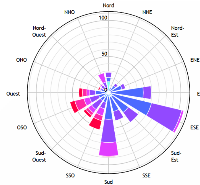
Figure 5. Rose des vents de la période de mesure
