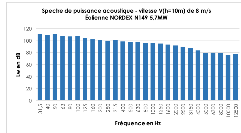
Figure 9. Graphique des niveaux de puissance acoustique d'une Nordex N149 - 5,7 MW (STE) par bande de tiers d'octave à la vitesse de 8 m/s (à la hauteur standardisée de 10 m)
