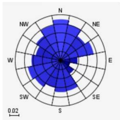
Figure 4. Rose des vents long terme
