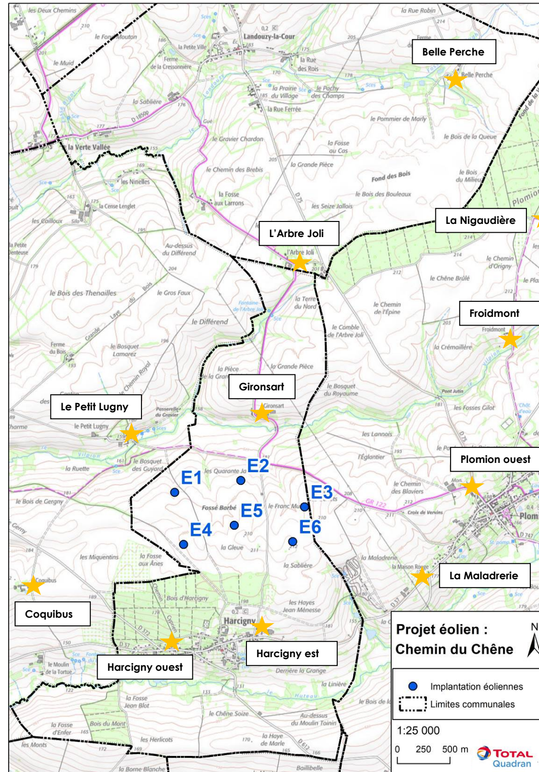
Figure 7. Implantation des points de contrôle et des éoliennes
